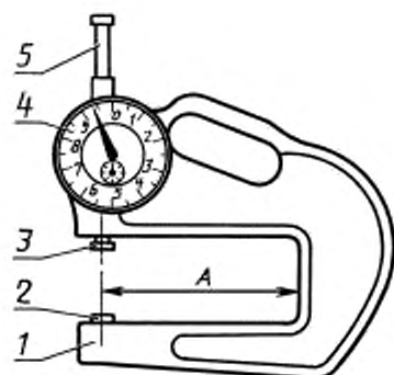
1 — корпус; 2 — пятка; 3 — измерительный наконечник; 4 — отчетное устройство; 5 — измерительный стержень; A — вылет
