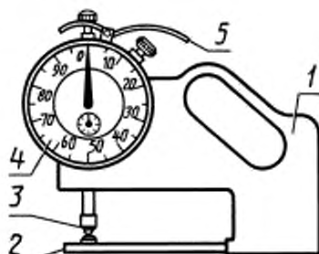
1 — корпус; 2 — неподвижный стержень; 3 — измерительный наконечник; 4 — отчетное устройство; 5 — арретир
