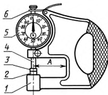
1 — корпус; 2 — пружина; 3 — измерительный наконечник; 4 — измерительный стержень; 5 — отсчетное устройство; 6 — арретир; А — вылет
